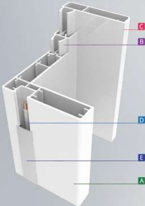
Door Frame Details
