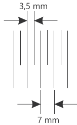
GA A Lamel Aralığı Fin Spacing
